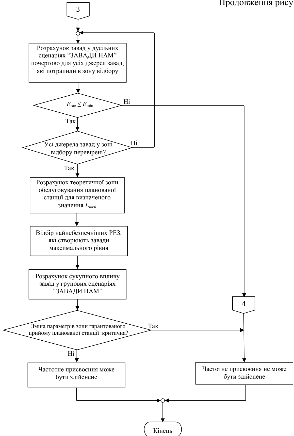
Рисунок — Схема проведення розрахунків EMC РЕЗ радіомовної служби під час здійснення нових частотних присвоєнь РЕЗ
